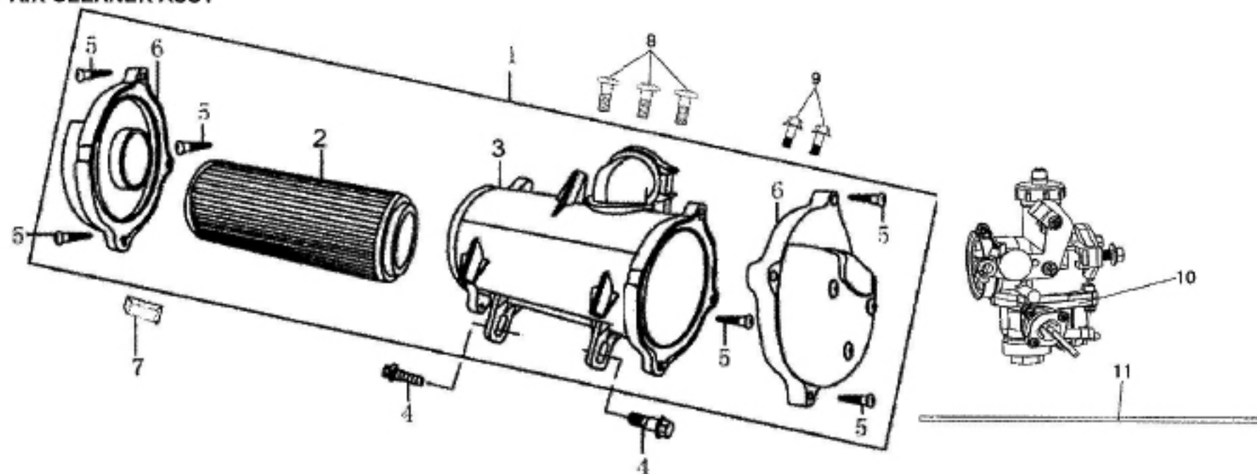
F-5 空滤器 AIR CLEANER ASSY
