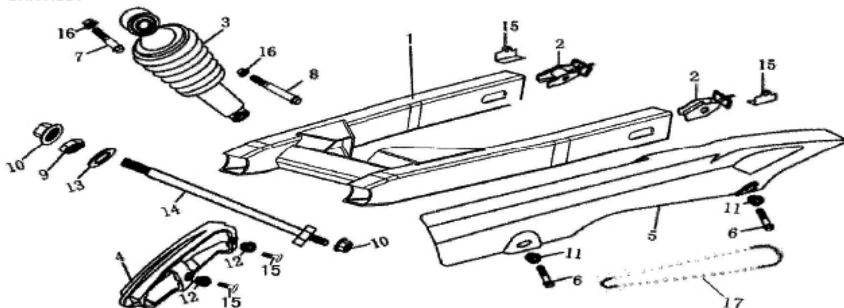
F-13 平叉总成 REAR FORK ASSY
