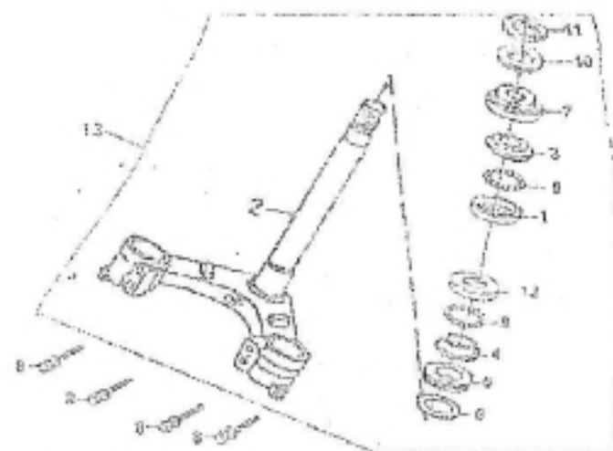
F-10 方向柱组合 STEERING STEM ASSY
