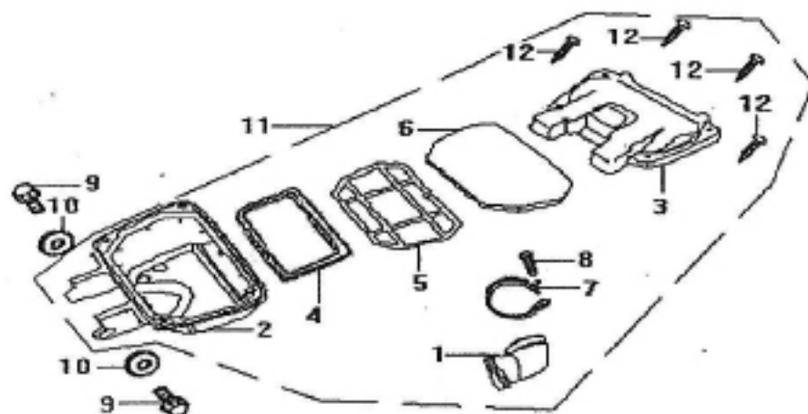
F-3 空滤器总成 AIR CLEANER ASSY
