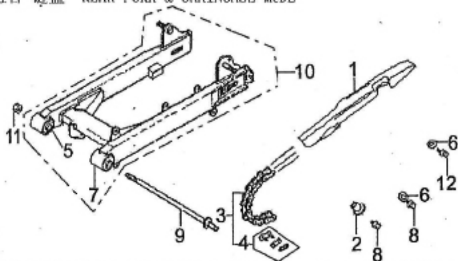
F-12 平叉焊接组合 链盒 REAR FORK & CHAINCASE MODE
