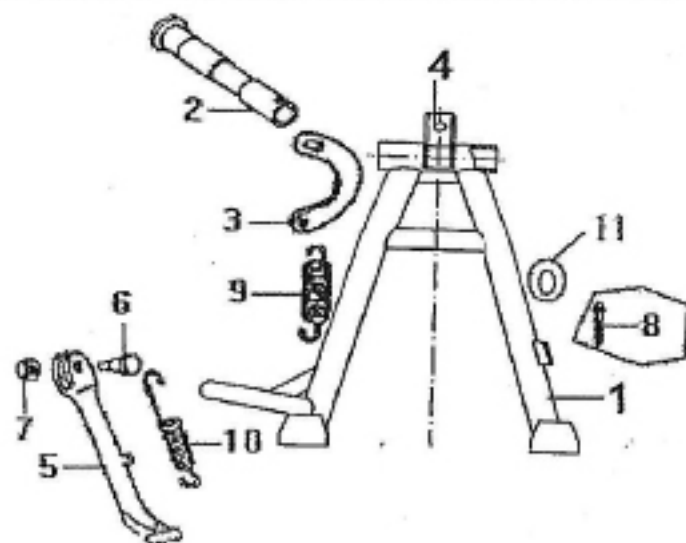
F-9 主支架 CENTER STAND
