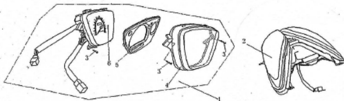
F-1 仪表及大灯 METER & HEADLIGHT
