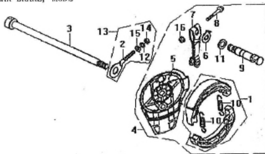
P-15 后制动器 REAR BRAKE, MODE
