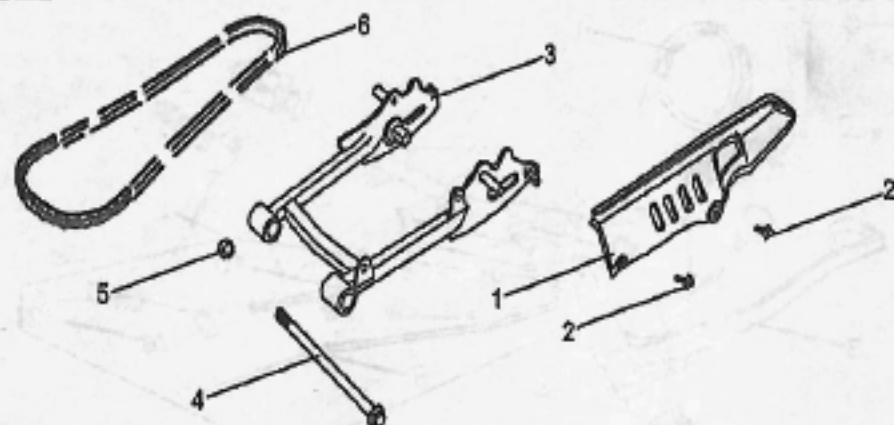
F-13 平叉焊接组合、链盒 REAR FORK WELDMENT & CHAINCASE
