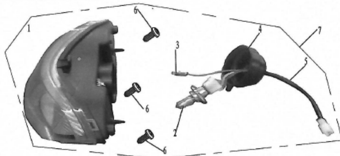
F-14 前大灯 Head Light
