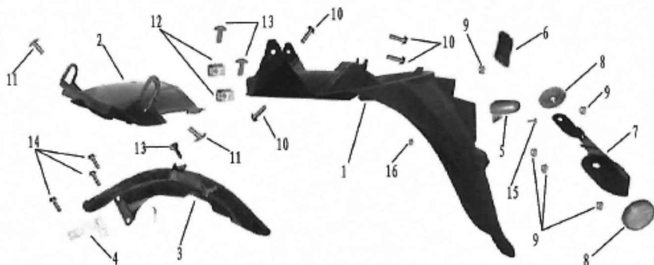
F-24 后挡泥板 REAR FENDER
